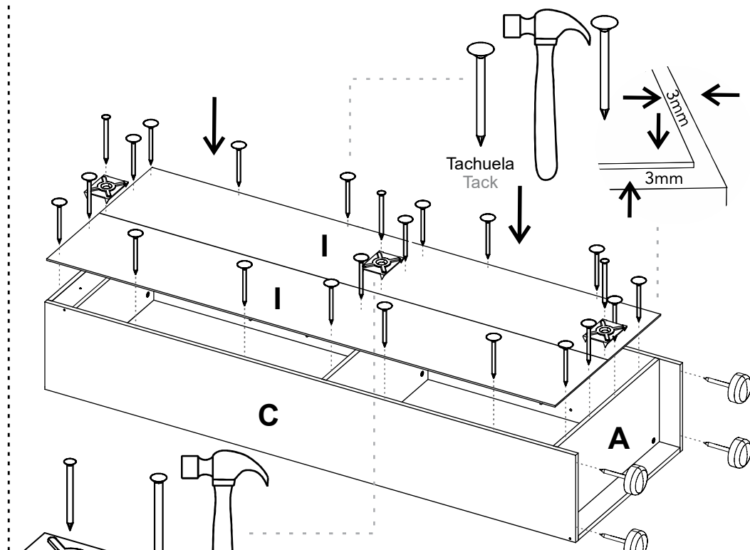
Puntilla Nail
